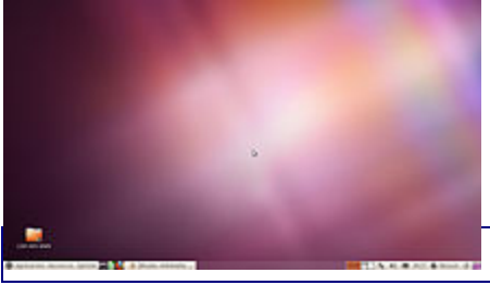
Ubuntu 11.04
